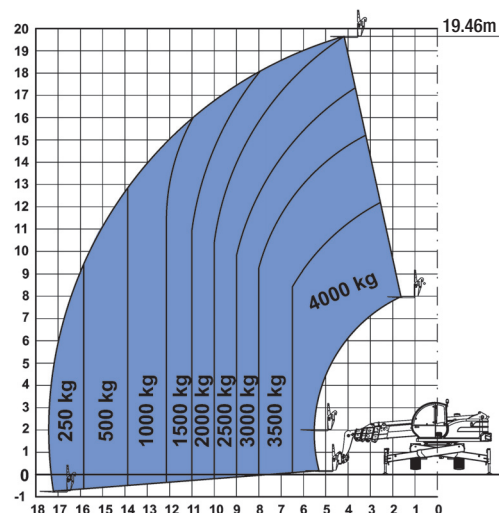
Diagramma di carico (con stabilizzatori) EN 1459, allegato B
